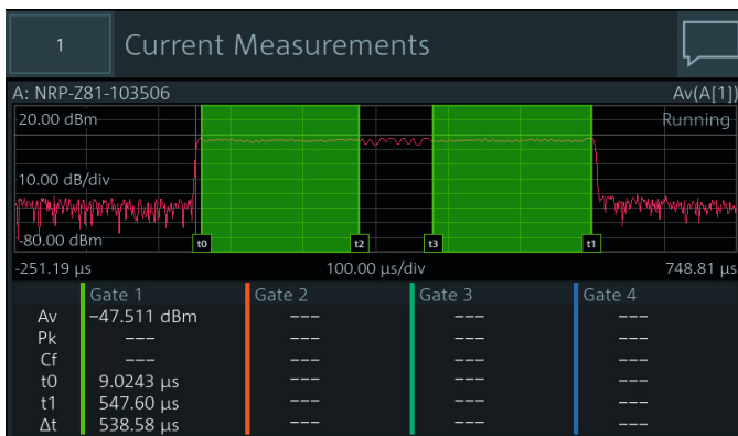
Определение мощности пакетного сигнала EDGE с помощью трехканального диодного датчика мощности R&S®NRPxxS(N) и функции стробирования; исключение тренировочной последовательности в центре сигнала
